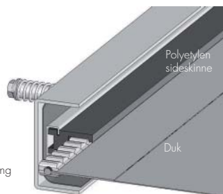
Snitt sideforsterkning
