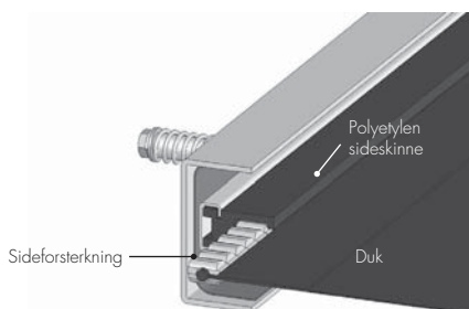
Snitt sideforsterkning
