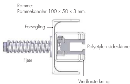
Snitt Sidskinne
